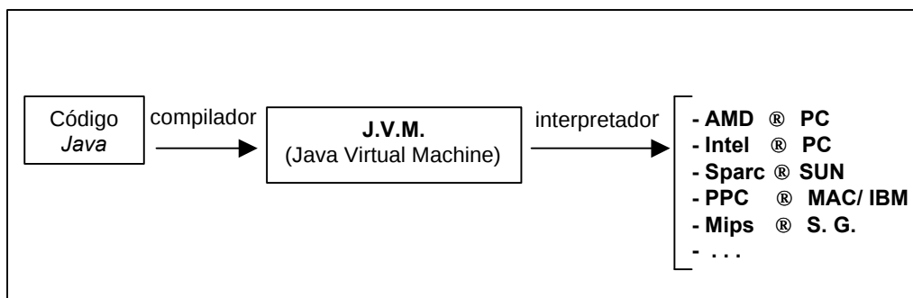
Figura 2.1: interpretação do código Java - O código Java é transformado em uma sequência de instruções que são interpretadas para o processador real da máquina.
